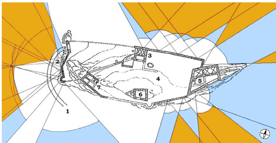
▲ Plán pokrytí hradu dělostřeleckou palbou, znázorňující nedostatky možnosti jeho obrany. Modře – pokrytí z jedné střílny, oranžově – křížová palba z více střílen, bíle – bez dělostřeleckého pokrytí. 1. přístupová cesta, 2. první obranná linie, 3. věžová brána, 4. nádvoří, 5. nový palác, 6. donjon, 7. starý palác. Plán hradu dle kresby D. Meclové.
